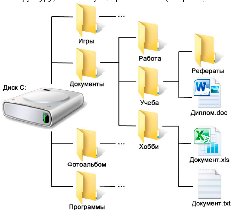
Рисунок 1. Дерево папок.
