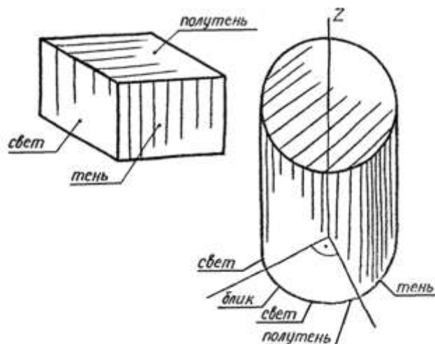
Рисунок 4 — Штриховка
